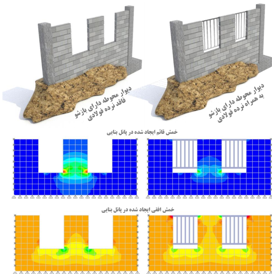
شکل ۵-۵- تاثیر نرده‌های فولادی باز شو در توزیع خمش خارج از صفحه پانل بنایی
