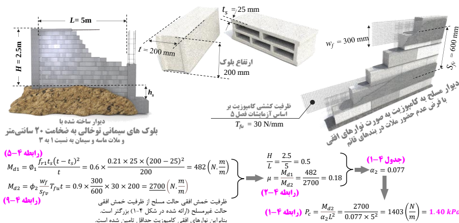
شکل ۴-۴- نمونه محاسبه ظرفیت خارج از صفحه برای یک پانل بنایی مسلح به کامپوزیت شبکه الیاف به صورت نوارهای افقی
