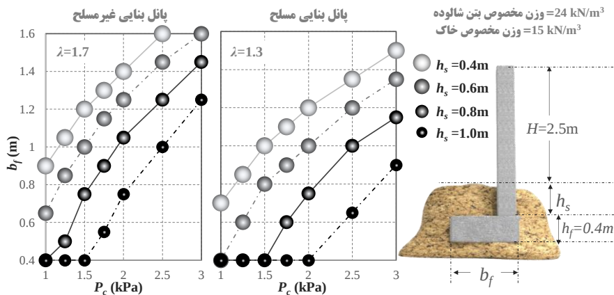
شکل ۴-۱۰- عرض مورد نیاز شالوده در صورتی که دیوار در لبه شالوده قرار دارد. در تمام موارد ارتفاع آزاد دیوار H=2.5m و عمق مقطع شالوده h_f=0.4m است.
