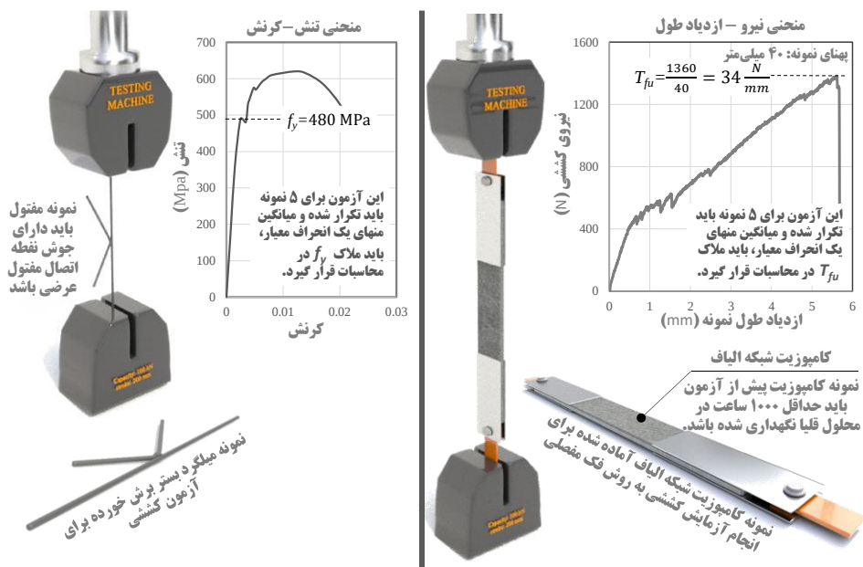
شکل ۵-۶- نحوه انجام آزمون‌های کششی میلگرد بستر و کامپوزیت شبکه الیاف
