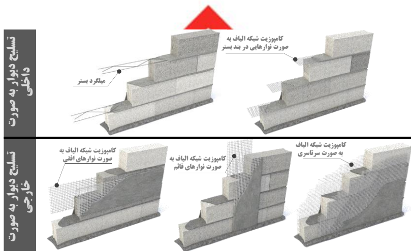
شکل ۲-۳- روش‌های تسلیح پانل بنایی به صورت داخلی و خارجی
