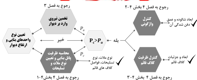
شکل ۲-۵- روند طراحی دیوارهای بنایی محوطه
