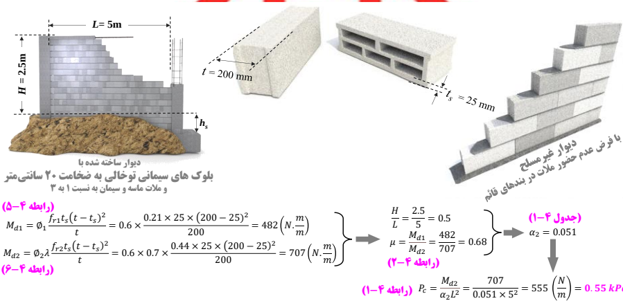
شکل ۱-۴ - نمونه محاسبه ظرفیت خارج از صفحه برای پانل بنایی غیرمسلح
