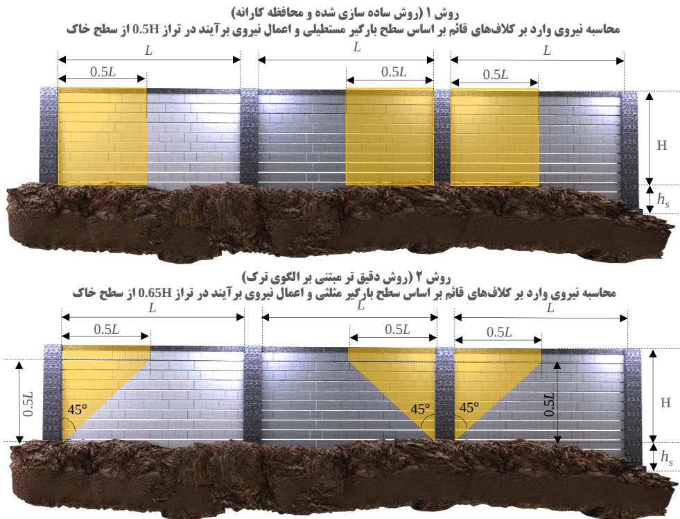
شکل ۱۲-۴ - محاسبه سطح بارگیر کلاف‌های قائم
