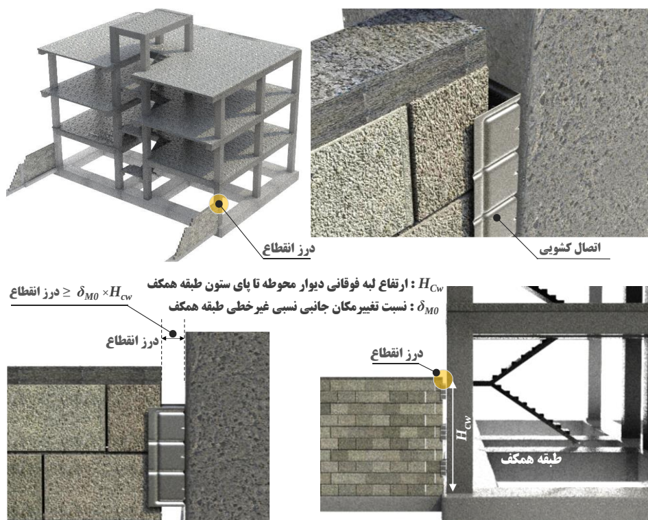
شکل ۵-۲- درز انقطاع مابین دیوار محوطه و ساختمان مجاور برای جلوگیری از آسیب به ستون سازه و دیوار محوطه
