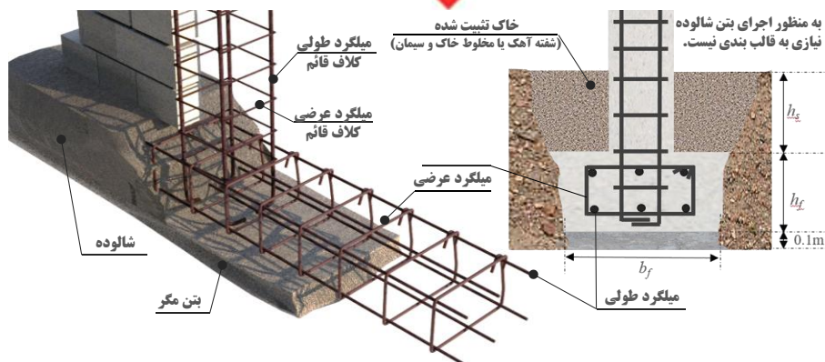
شکل ۴-۱۱- جزئیات اجرا و میلگردگذاری شالوده
