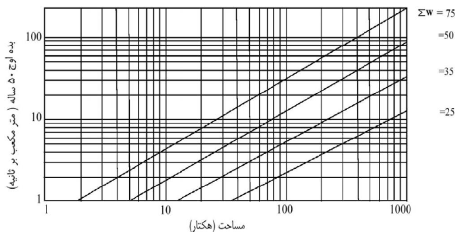
شکل ۷-۵- نمودار بر آورد سیلاب ۵۰ ساله ( Q_{50} ) به کمک مساحت حوضه (هکتار) و ضریب کوک ( W )
