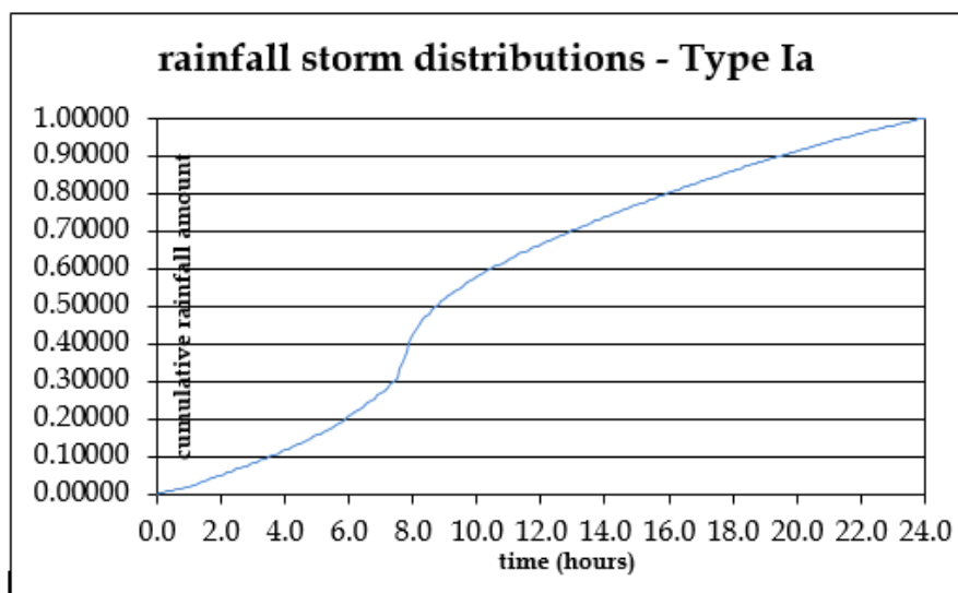
شکل ۸-۲- هایئوگراف Type Ia (SCS)
