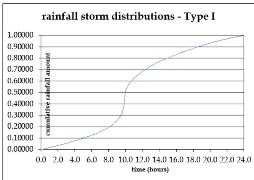
شکل ۸-۱- هایئوگراف Type I (SCS)
