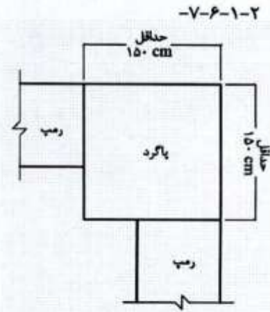
(ب) رمپ با تغییر مسیر
