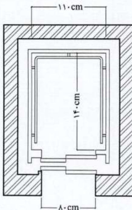
شکل شماره ۶۲: ابعاد داخلی اتاق آسانسور
